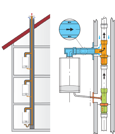
Slika 1. Sanacija jednokanalnog dimnjaka.
